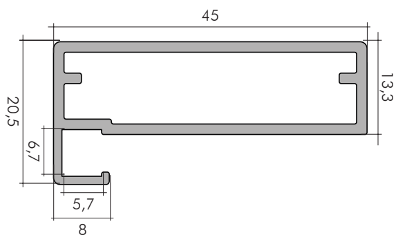
Guarnizione / Gasket 020057.L250.44
