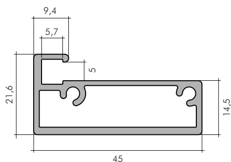
Guarnizione / Gasket 020057.L250.44
