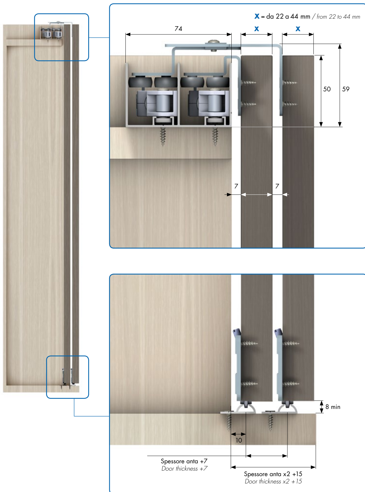
Sezione vista laterale Side view section
