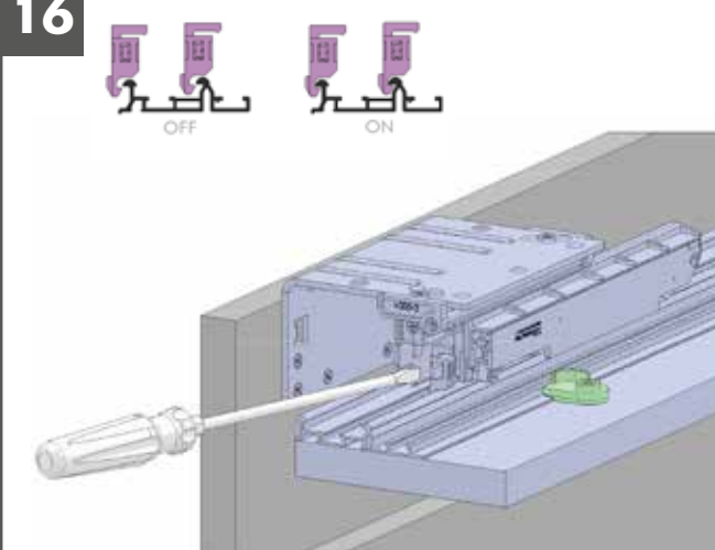
Anti scarrucolamento ante Anti derailment safety device
