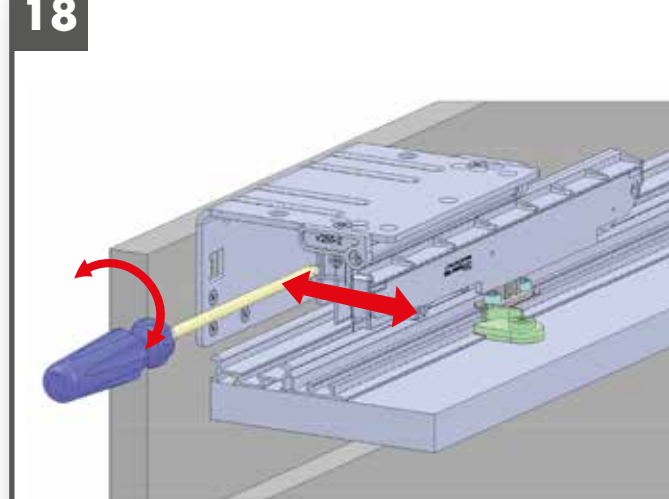
Regolazione assiale ante Axial adjustment doors
