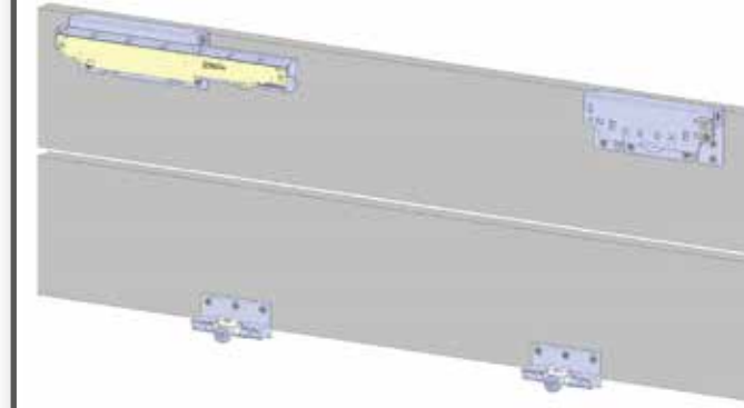
Anta interna SX Right internal door
