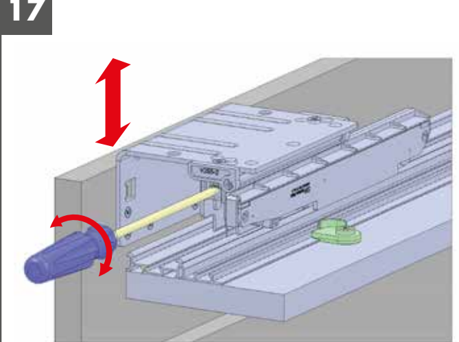
Regolazione verticale ante Vertical adjustment doors
