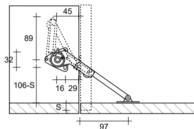
Applicazione anta legno
