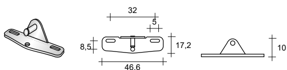
Applicazione anta alluminio
